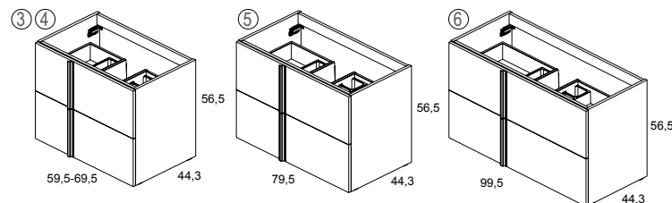
ONIX Opción Cajones Drawers Option
