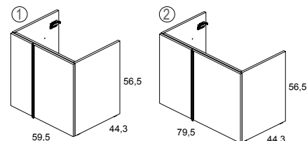
ONIX Opción Puertas Doors Option
