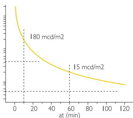
Curva de atenuación del mosaico STARLIGHT* Attenuation curve of the STARLIGHT* mosaic.
